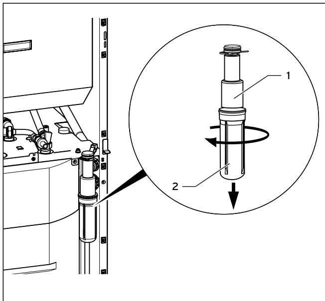
Рис. 8.8 Очистка сифона
