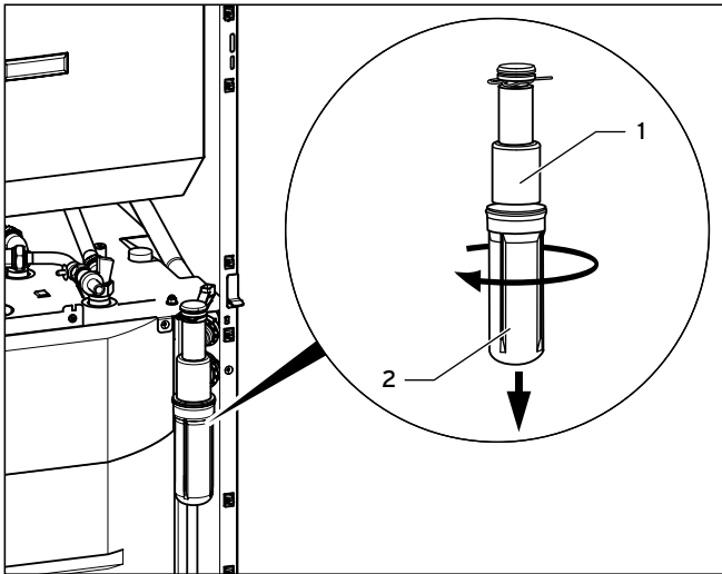
Рис. 6.2 Заполнение сифона
