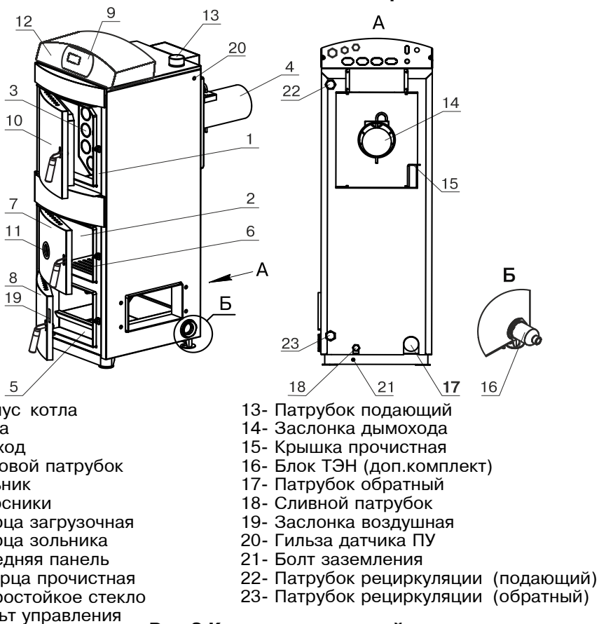
Рис.2 Котел отопительный
