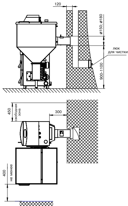
Рис.6 Схема установки котла
