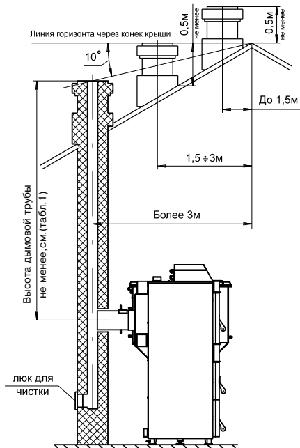
Рис.7 Варианты установки дымовой трубы
