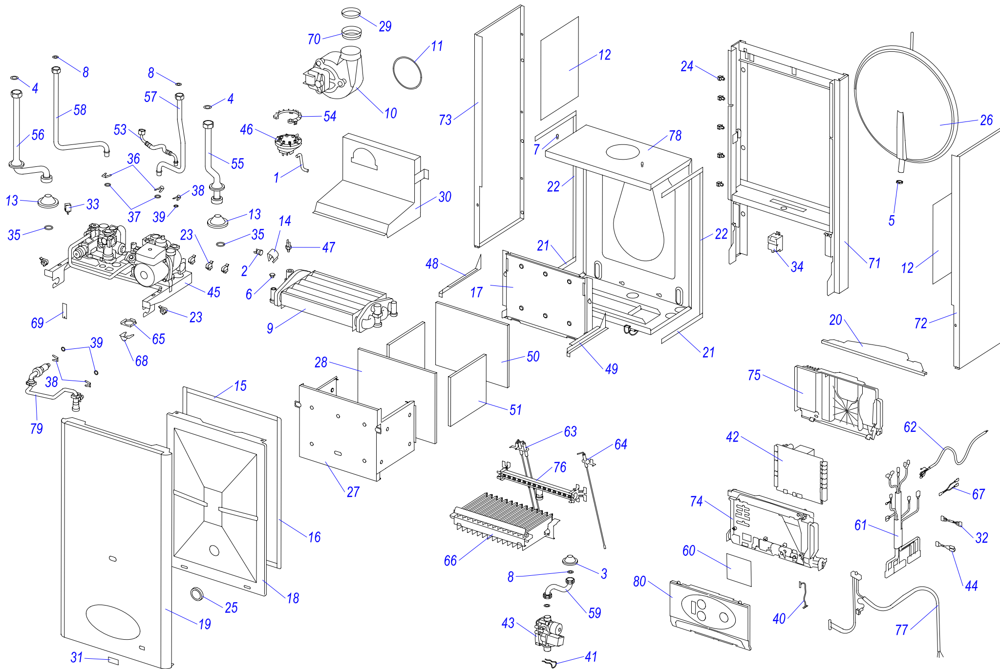
Навесные котлы
