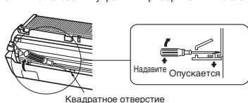
Квадратное отверстие
