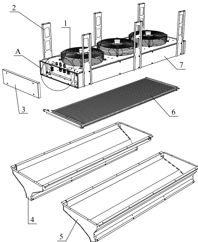
Рисунок 2. Воздушно-тепловая завеса
