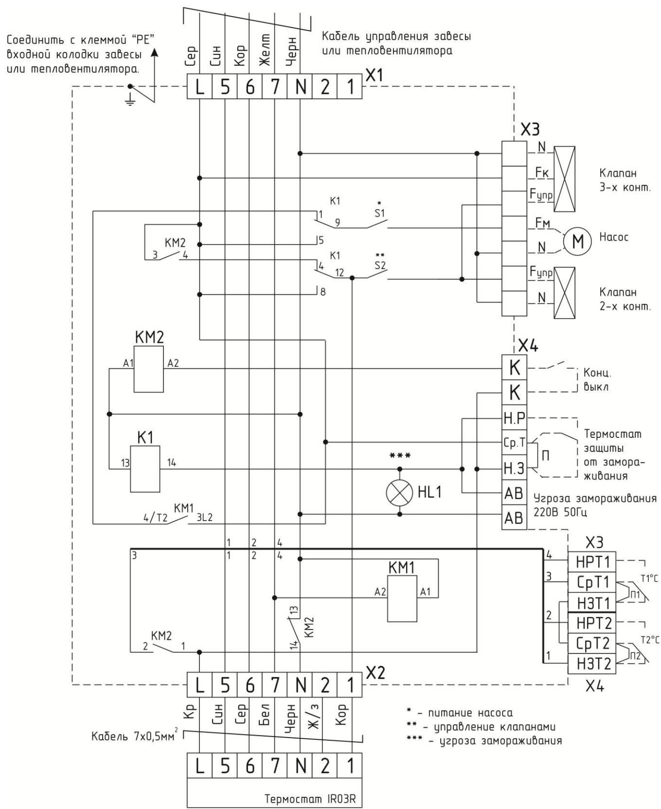
Рисунок 11-Электрическая схема подключения концевого выключателя, смесительного узла и термостата защиты от замораживания к занавесам и тепловентиляторам с водяным источником тепла и без источника тепла «Блок-W».
