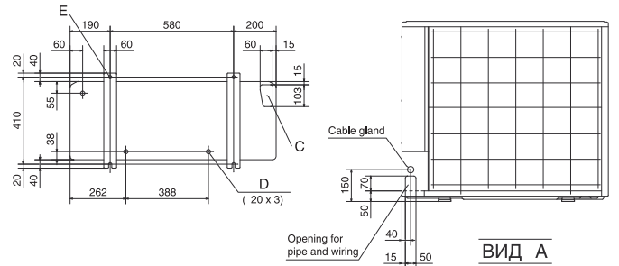
Минимальное пространство для установки 3HP
