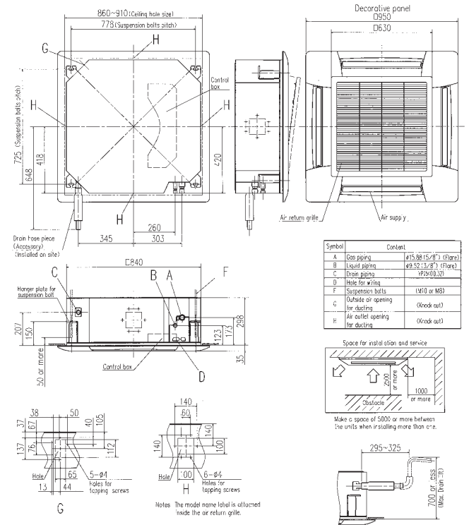
Модель FDT100VF, 125VF, 140VF1
