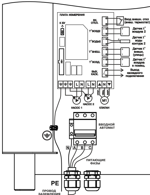
Рис.3 Схема подключения электроводонагревателя
