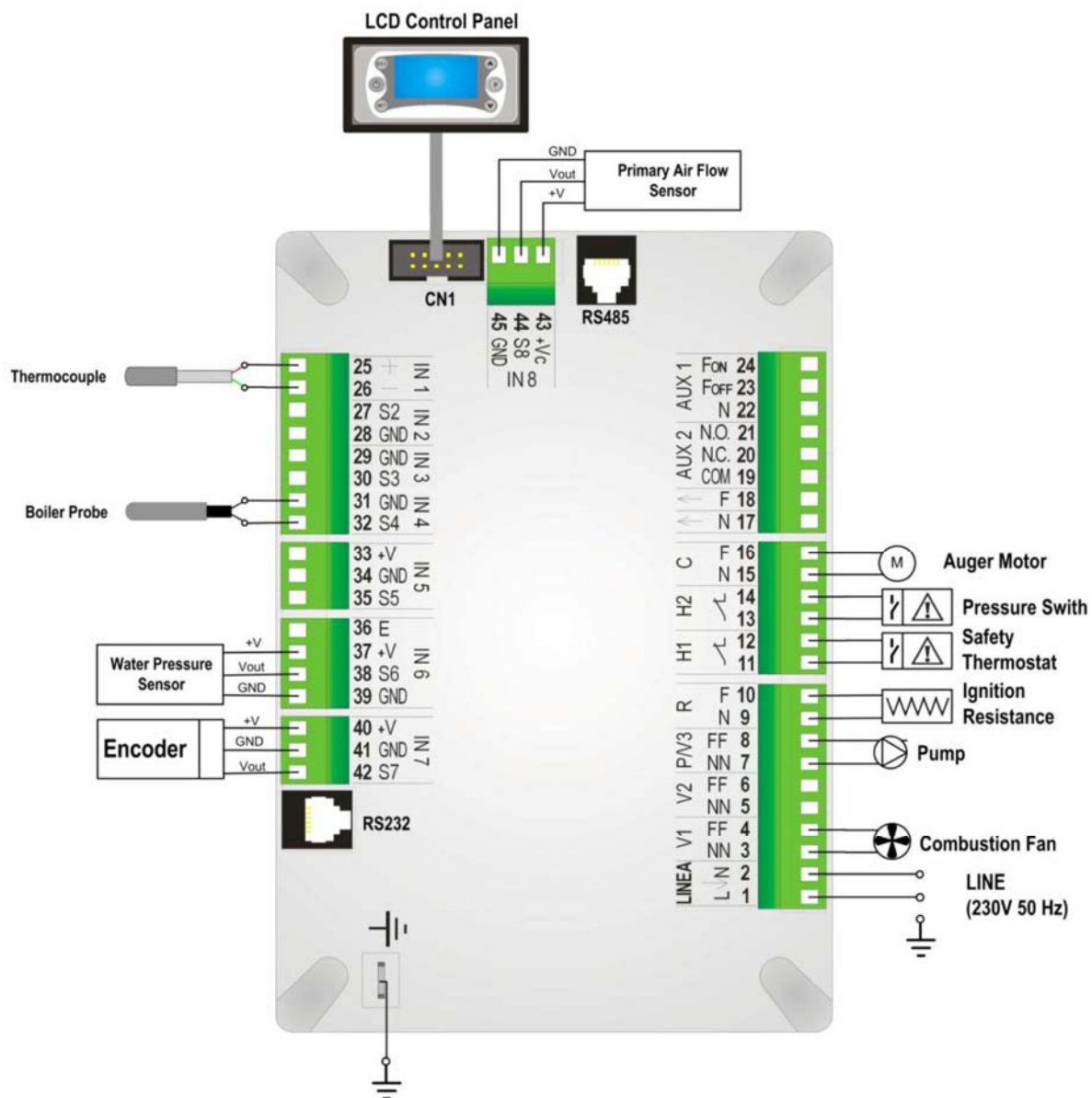
Рис 10. Электрические подключения
